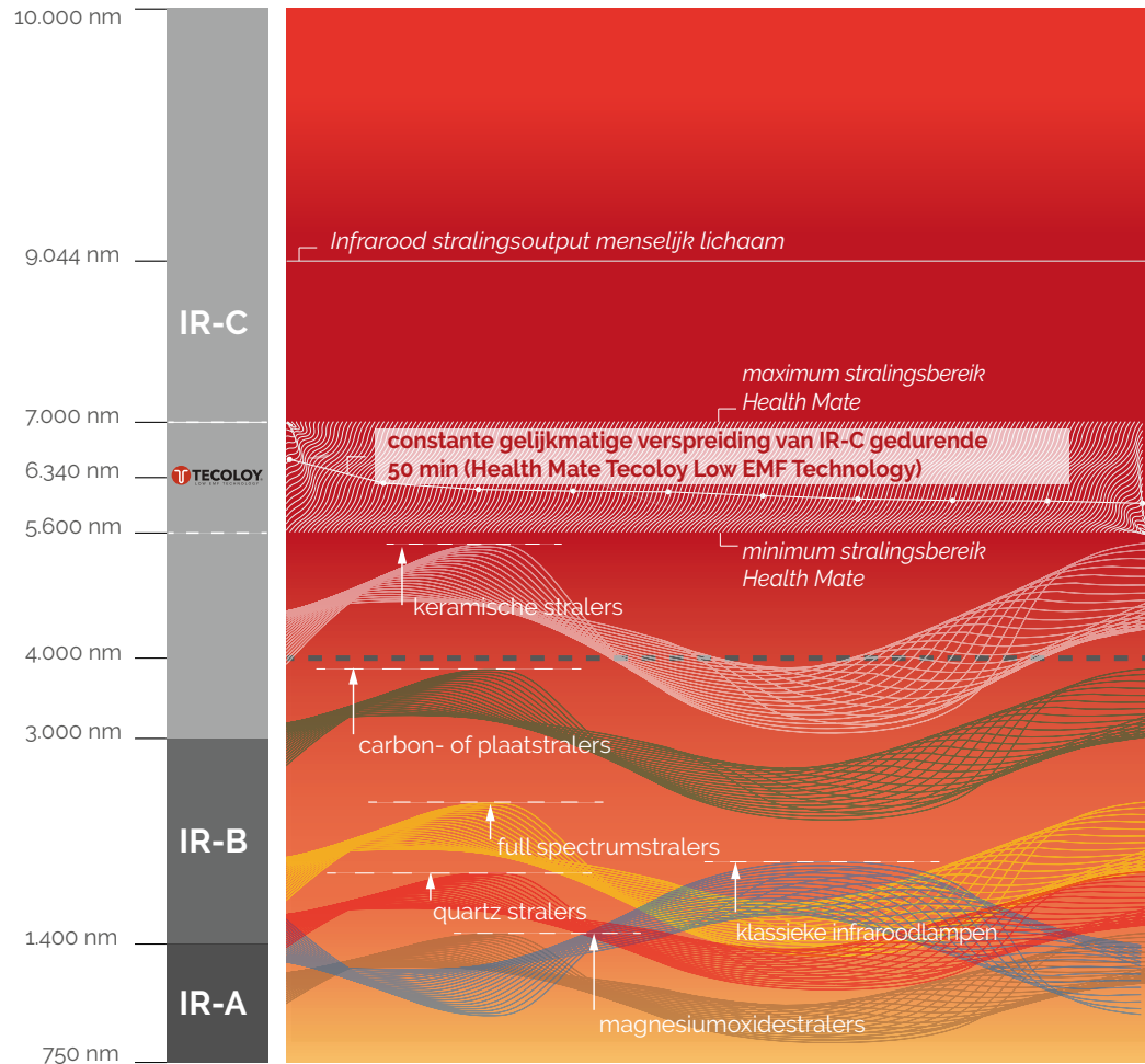
Spectrale emissies bij een constant maximaal stralingsvermogen
